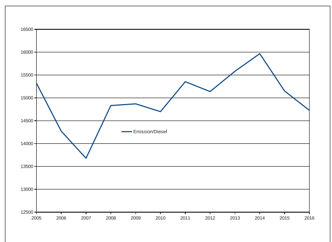
Abb. 1b: Entwicklung spezifische NO x -Emission als Gramm NO 2 je Diesel-Pkw und Jahr
